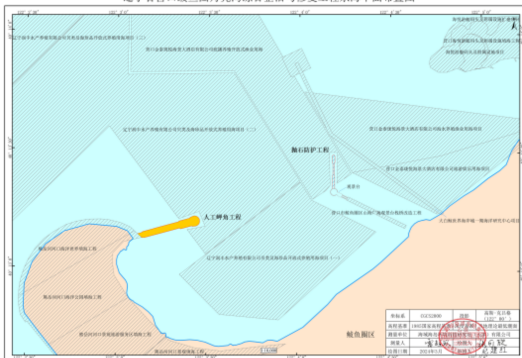
辽宁省营口鲅鱼圈月亮湾综合整治与修复工程宗海平面布置图
