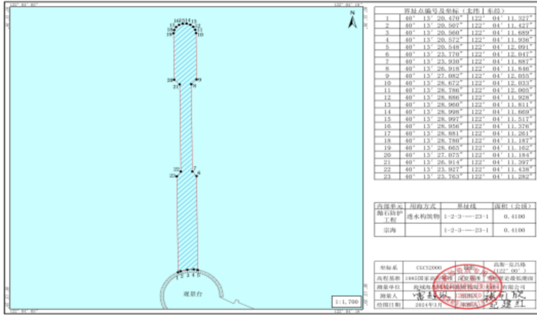
辽宁省营口鲅鱼圈月亮湾综合整治与修复工程宗海位置图
