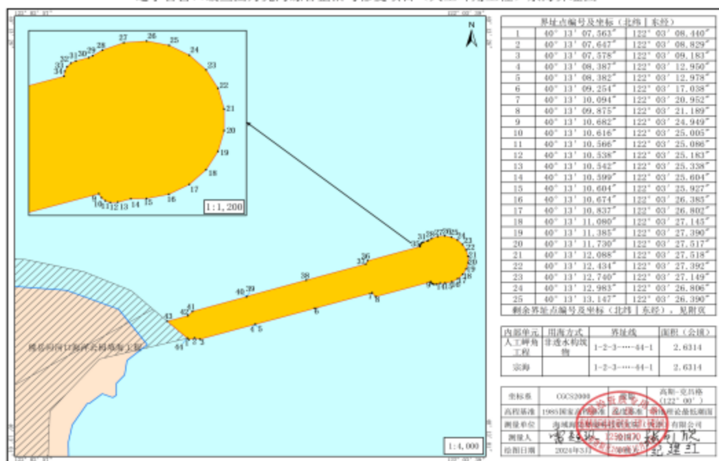
辽宁省营口鲅鱼圈月亮湾综合整治与修复项目(人工岬角工程)宗海界址图
