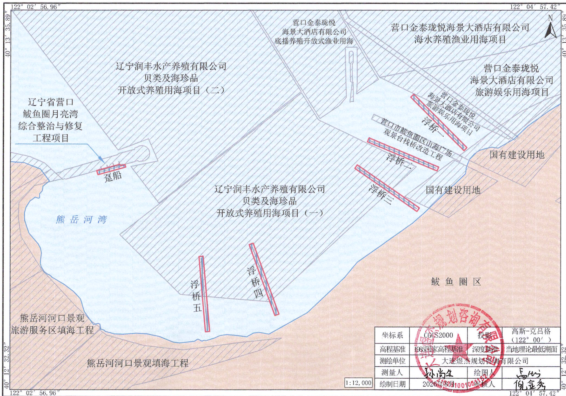
营口文化旅游产业集团有限公司海上看营口项目宗海平面布置图
