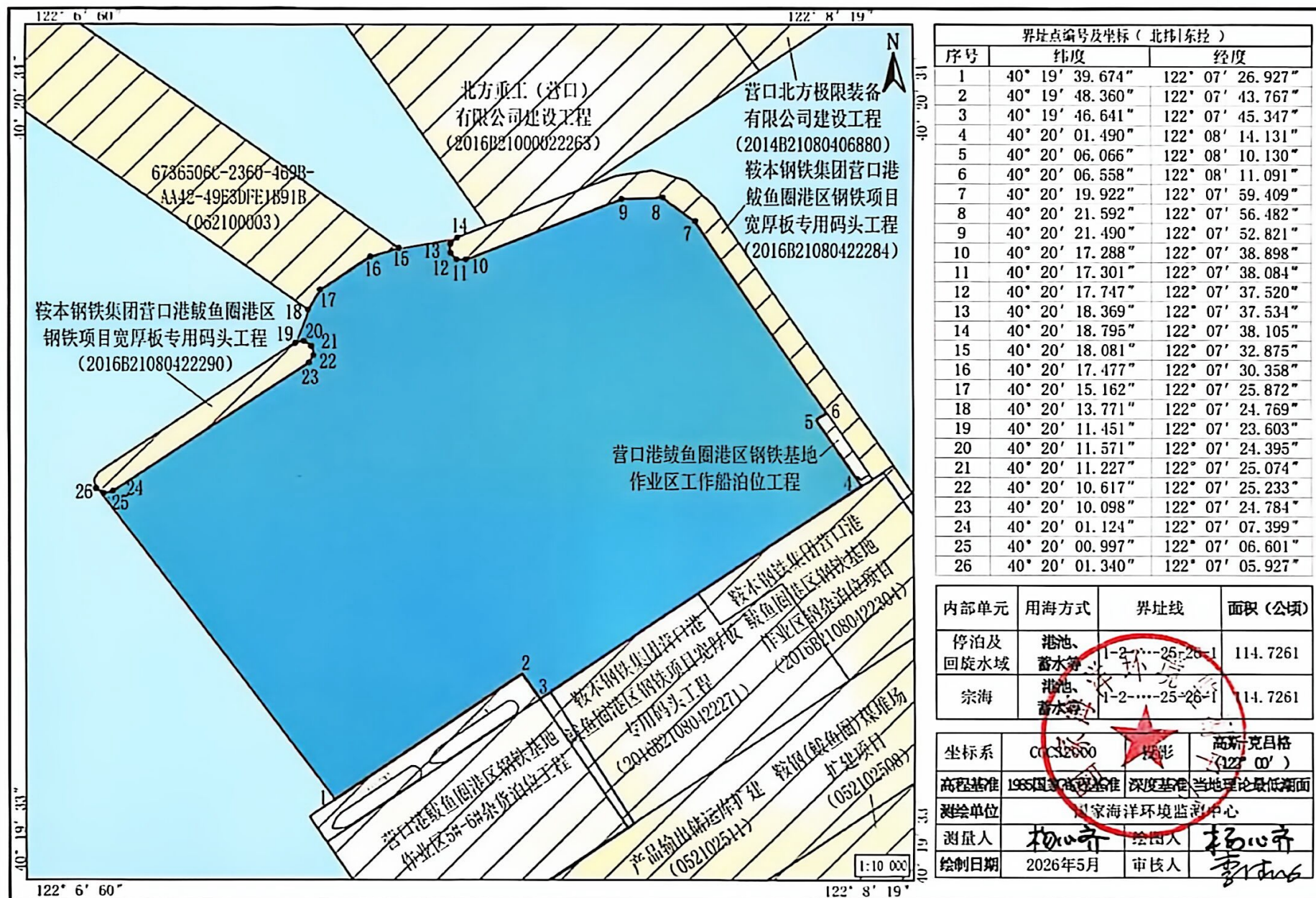
鞍山钢铁集团公司鲅鱼圈钢铁项目专用码头（港池）项目宗海界址图
