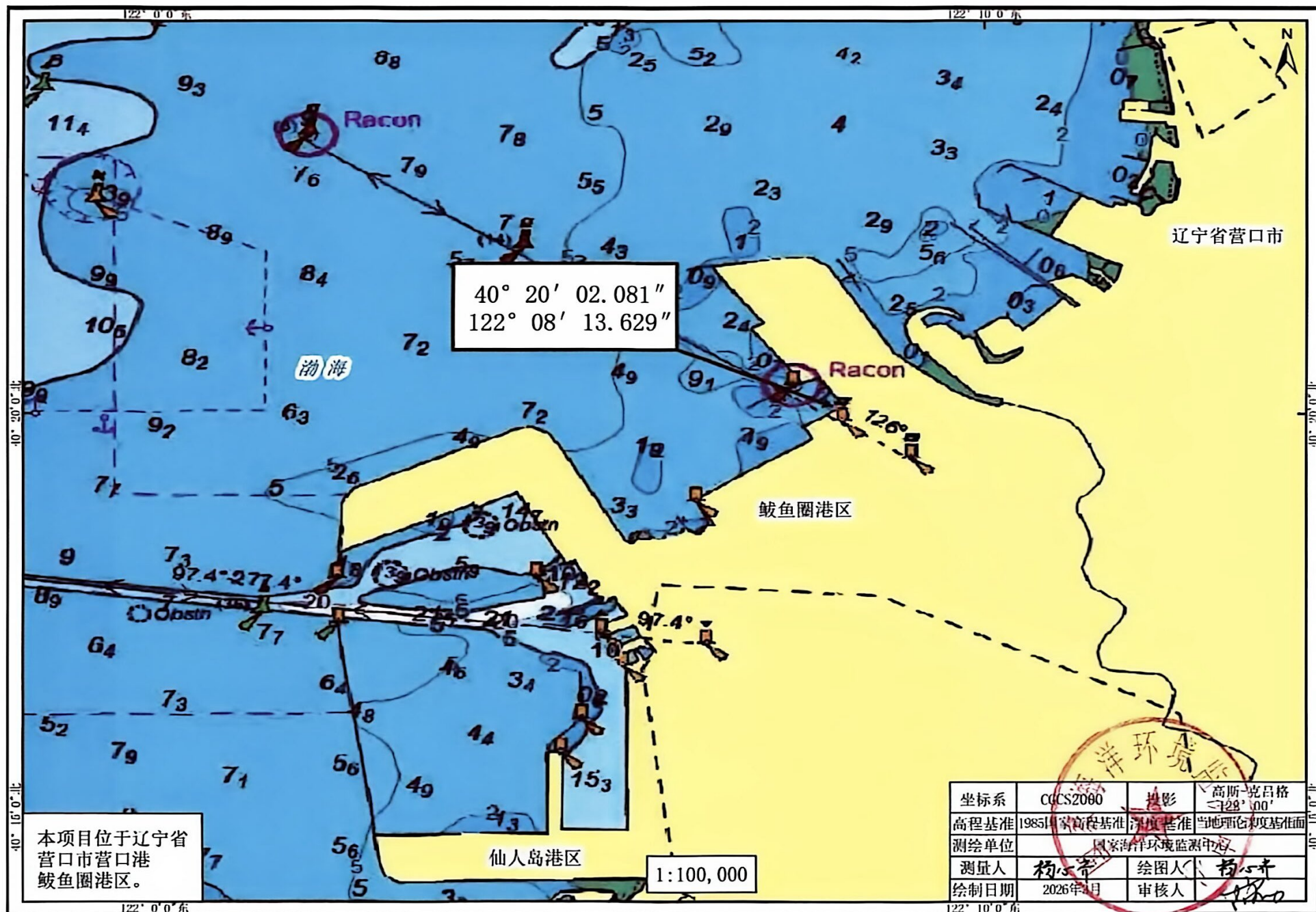
营口港鲅鱼圈港区钢铁基地作业区工作船泊位工程宗海位置图
