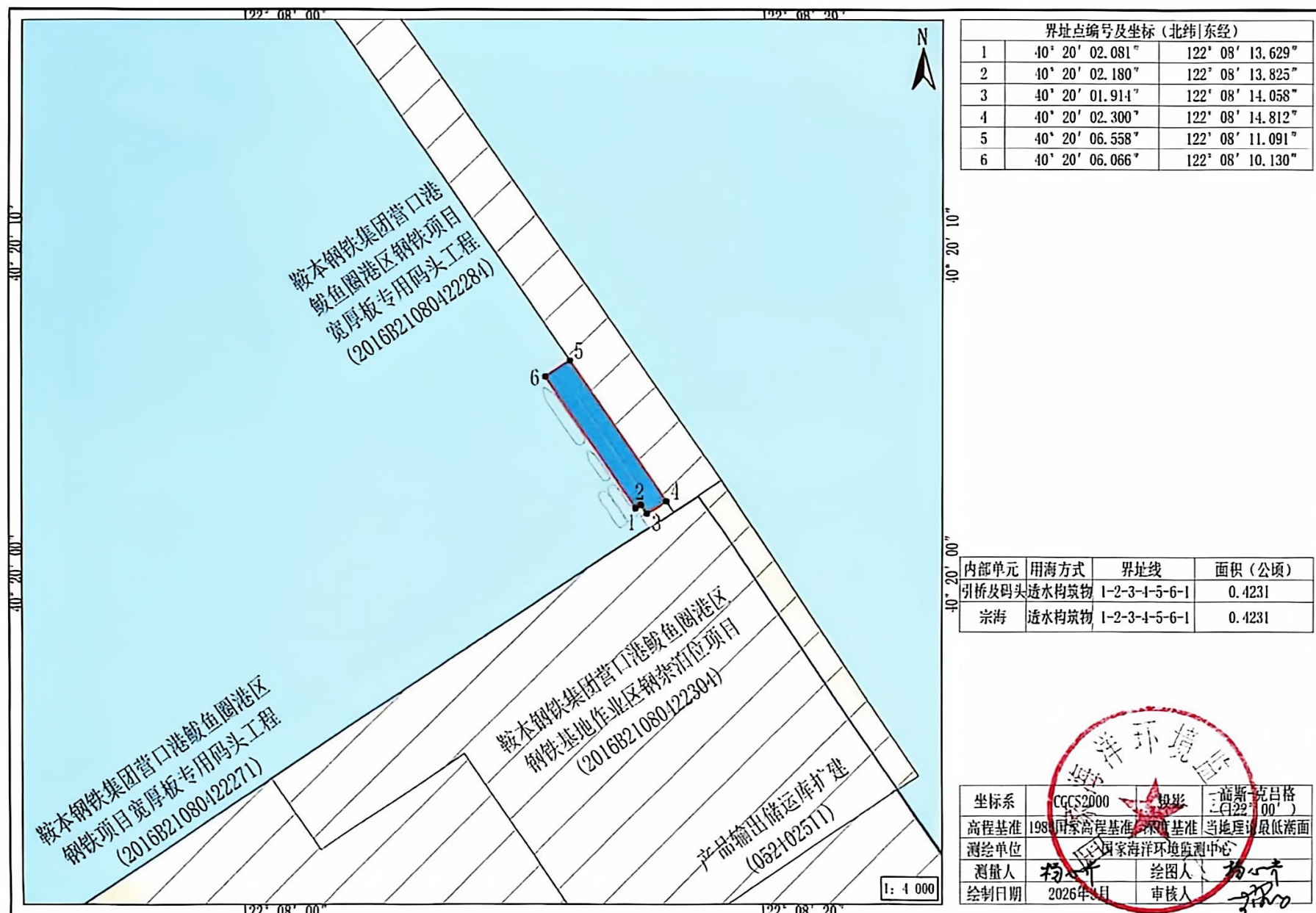
营口港鲅鱼圈港区钢铁基地作业区工作船舶泊位工程宗海界址图
